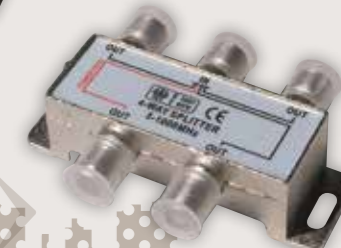
R011 Rozbočovač 4xF 4x7,0dB / 500MHz ret.>20dB 1xDC
